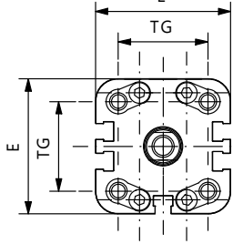
Ø32
