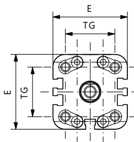
Ø32
