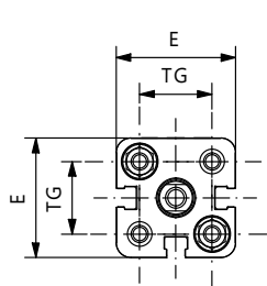
Ø20 - Ø25
