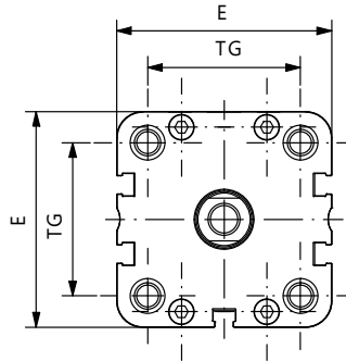
Ø40 - Ø50
